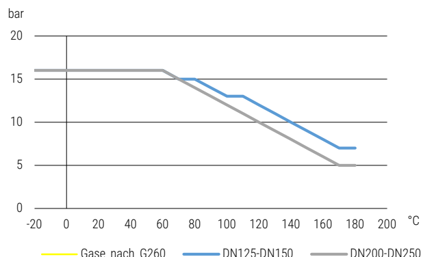
Druck-Temperatur-Diagramm pressure-temperature-diagram
